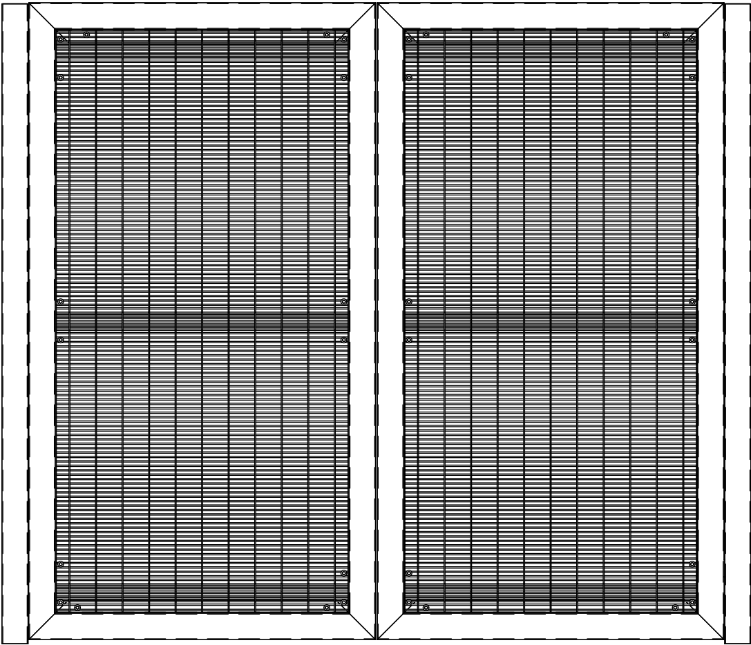
2 BACK ELEVATION 1 : 15
