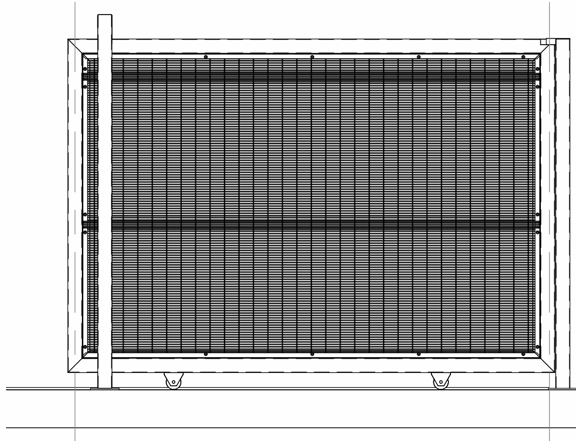
2 BACK ELEVATION 1 : 20
